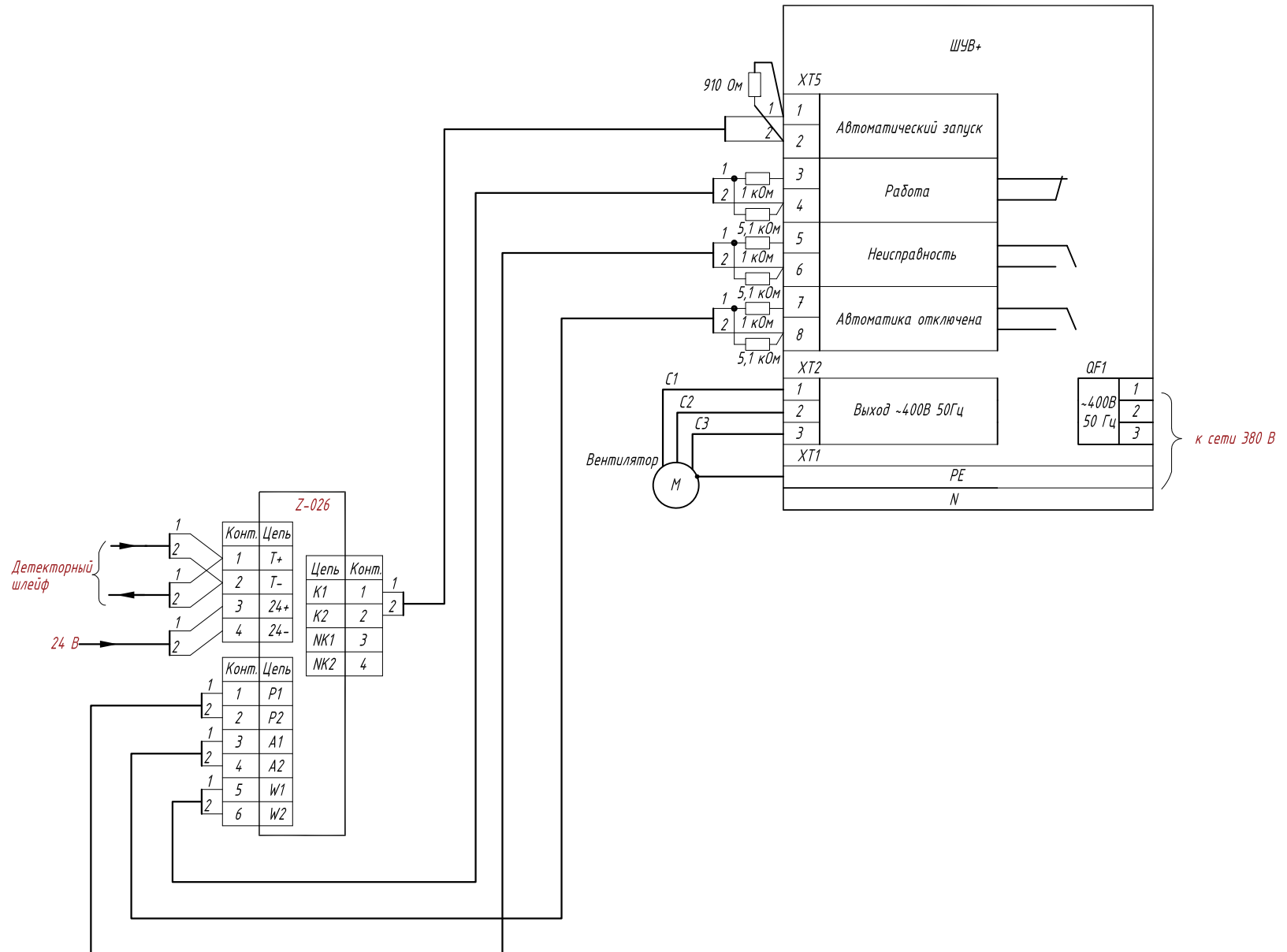
Схема подключения шкафа управления вентиляторами противодымной защиты серии ШУ типа ШУВ+. Схема внешних подключений для управления одним вентилятором 380В.
